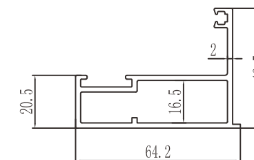
ZYMQ26026 1.094 kg/m
