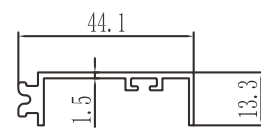
ZYMQ26027 0.358 kg/m
